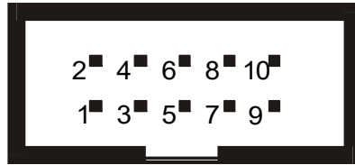
プログラマーの ISP コネクタの正面
